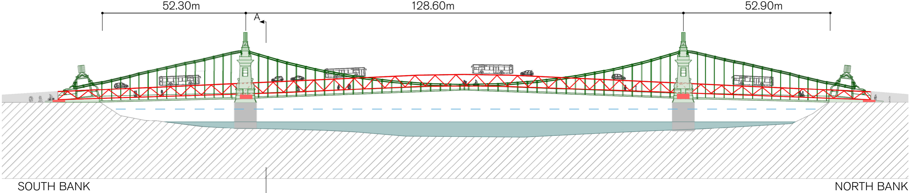
Elevation
